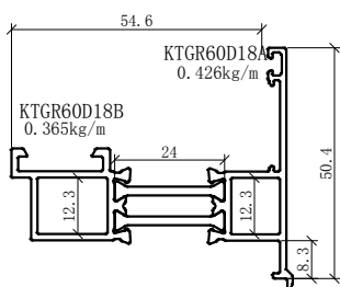
配KTGR60D04角码
