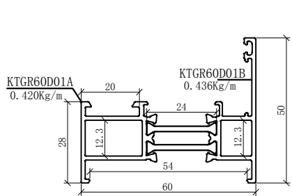
配KTGR60D04角码
