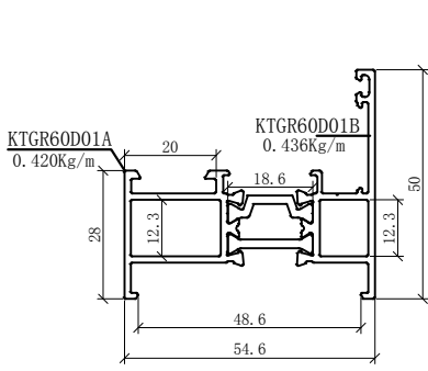
配KTGR60D04角码
