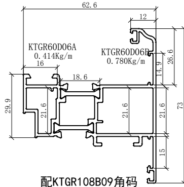
配KTGR108B09角码
