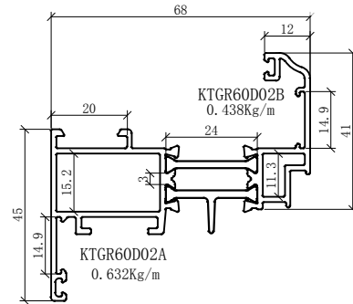
配KTZJ50A16+KTJM05角码
